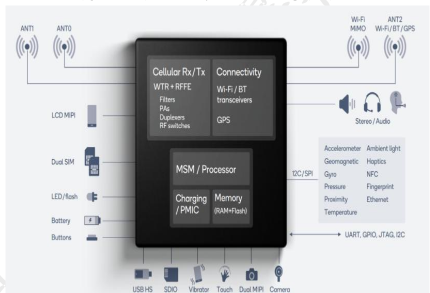
圖三、高通(Qualcomm)發展之 System-in-Package(SiP)封裝
