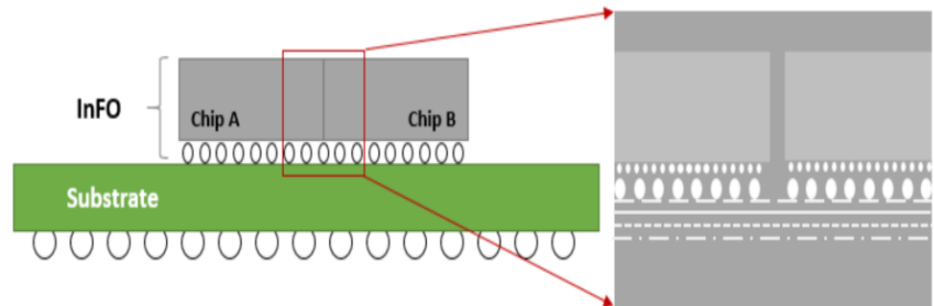
圖二、台灣半導體晶圓代工廠發展之 Info-on-Substrate(InFO-oS)
